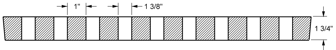
SECTION A-A
