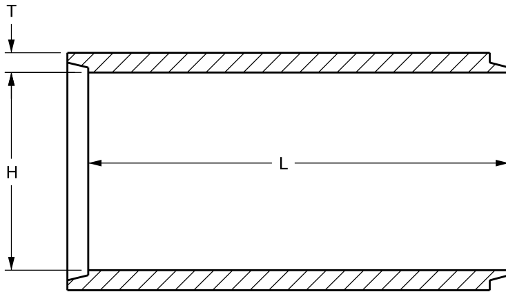
LONGITUDINAL SECTION
