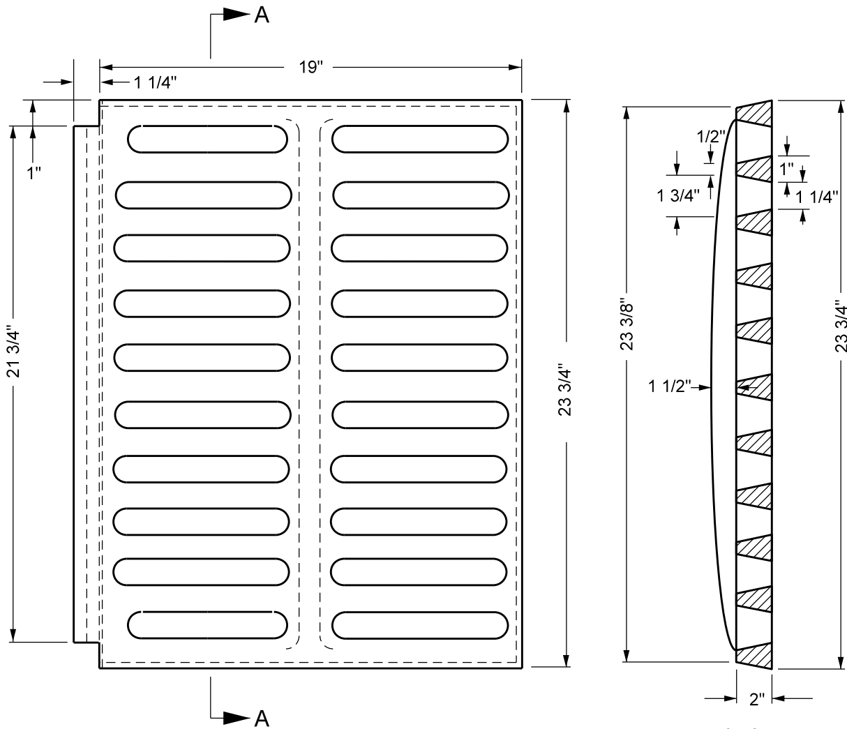
A - A
