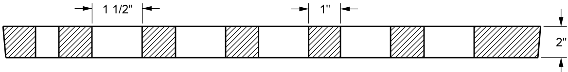
SECTION A-A
