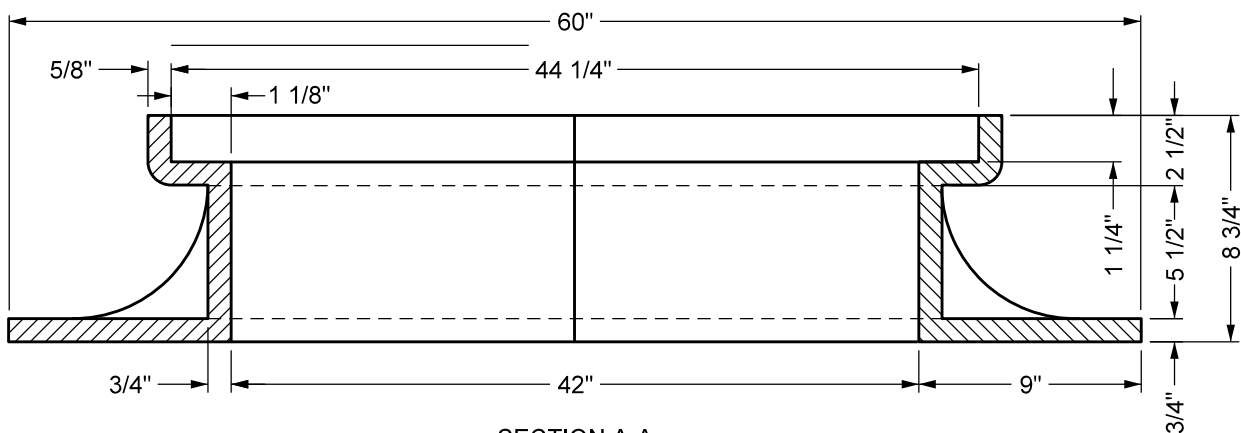
SECTION A-A
